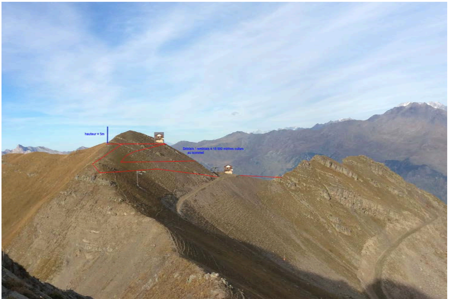
Travaux envisagés sur les crêtes, à la Pointe des Chaudannes, côté Karellis (déblais de 18 000 mètres cubes au sommet arasé et création d'une plateforme
