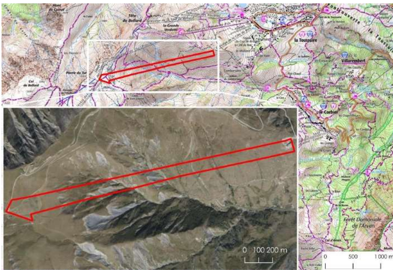
Figure 2: Localisation de la zone d'étude dans la combe de Comborsière
